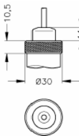
Кабельный штепсель (IP 68) 7
