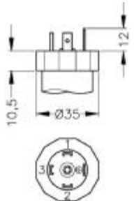
DIN 43650 (IP 65)
